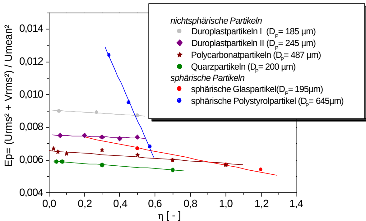
Abbildung 5-29: Normierte Energie der Partikelschwankungsgeschwindigkeit in Abhängigkeit von der Beladung für unterschiedliche Partikelgrößen und -formen. Wand- rauhigkeit R_0 , U_{\text{mittel}} zwischen 19,8 und 20,2 m/s.
