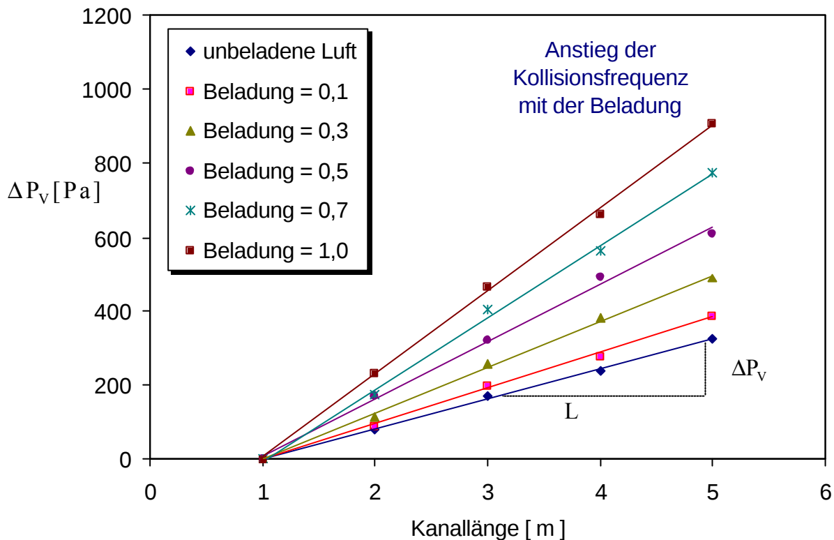
Abbildung 5-46: Druckverlust in Abhängigkeit von der Kanallänge, Wandrauhigkeit R_0 , D_p = 195 \mu\text{m} - Glaspartikeln. Normiert auf den Anfangsmesswert bei Kanallänge 1m, U_{\text{mittel}} = 20 \text{ m/s} .
