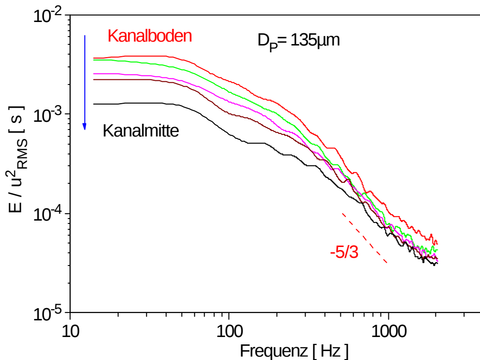
Abbildung 5-40: Energiespektren für unterschiedliche Abstände ( \Delta H = 3,5 \text{ mm} ) vom Kanalboden. D_p = 135 \mu\text{m} , Wandrauhigkeit R0, U_{\text{mittel}} = 20,2 \text{ m/s} , \eta = 1,0
