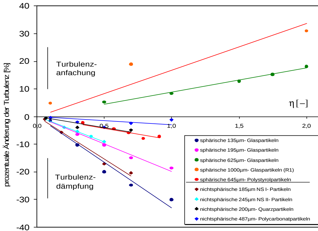
Abbildung 5-36: Turbulenzmodifikation in Abhängigkeit von der Beladung für unterschiedliche Partikelarten. U_{\text{mittel}} zwischen 19,9 und 20,2 m/s, Wandrauhigkeit R0.
