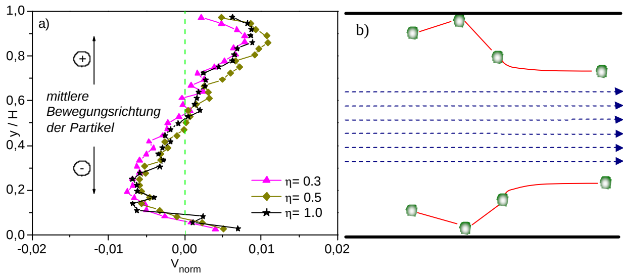
Abbildung 5-10: a) Normiertes vertikales Profil der mittleren vertikalen Geschwindigkeitskomponente der 100µm- Partikeln bei einem U_{\text{mittel}} von 19,7 m/s und der Wandrauhigkeit R2, b) Schematische Darstellung des Bewegungsverlaufes eines Partikels vor und nach einer Wandkollision.
