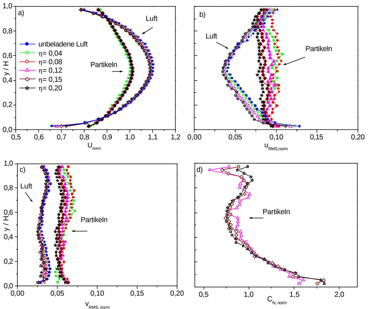
Abbildung 5-13: a-c) Normierte vertikale Profile der Luft und der 60 µm Partikel bei einem U_{\text{mittel}} von 19,7 m/s und der Wandrauhigkeit R2: a) horizontale Geschwindigkeit der Luft und der Partikel, b) RMS- Profile der horizontalen Komponenten, c) RMS- Profile der vertikalen Komponenten, d) Profil der normierte vertikalen Anzahlkonzentration der Partikel.
