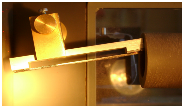
Abbildung 4-7: a), b) Versuchsstand mit Kamera für die Analyse der Wandkollision sphärischer und nichtsphärischer Partikeln.
