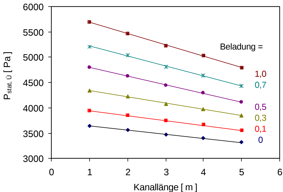
Abbildung 5-45: Statischer Überdruck entlang des Kanals für unterschiedliche Beladungen, Wandrauhigkeit R0, D_p = 195\mu\text{m} - Glaspartikeln, U_{\text{mittel}} = 20 \text{ m/s} .
