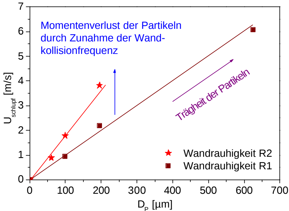
Abbildung 5-16: Änderung der Schlupfgeschwindigkeit in Abhängigkeit von der Partikelgröße und der Wandrauhigkeit bei einer Beladung von 0,1 (bei 625 \mu\text{m} Partikeln \eta=1 )
