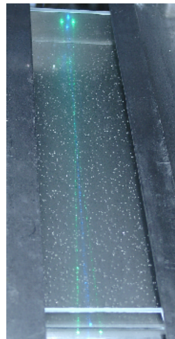
Abbildung 4-20: Mit 625µm- Partikeln beladene Kanalströmung.
