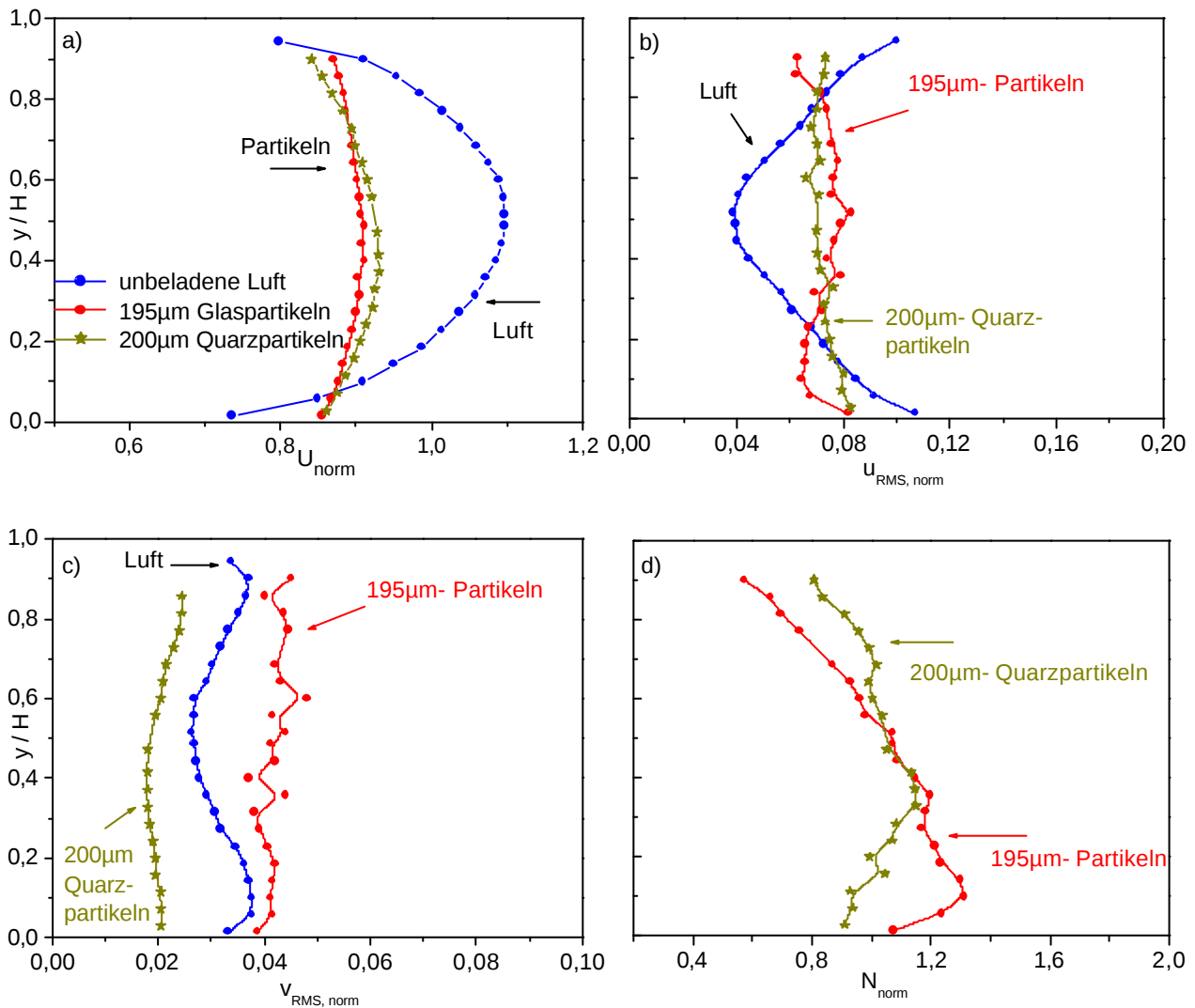
Abbildung 5-28: Normierte Profile der sphärischen 195µm- Glaspartikeln und der nichtsphärischen Quarzpartikeln bei einer Beladung von \eta = 0,3 , einem U_{\text{mittel}} von 20,2 m/s ( D_p = 195\mu\text{m} ) und U_{\text{mittel}} = 20,1 m/s ( D_p = 200\mu\text{m} ) und der Wandrauhigkeit R0: a) horizontale Geschwindigkeit der Partikeln, b) RMS- Profil der horizontalen Schwankungsgeschwindigkeit, c) RMS- Profil der vertikalen Schwankungsgeschwindigkeit, d) vertikale Sampleverteilung der Partikeln.
