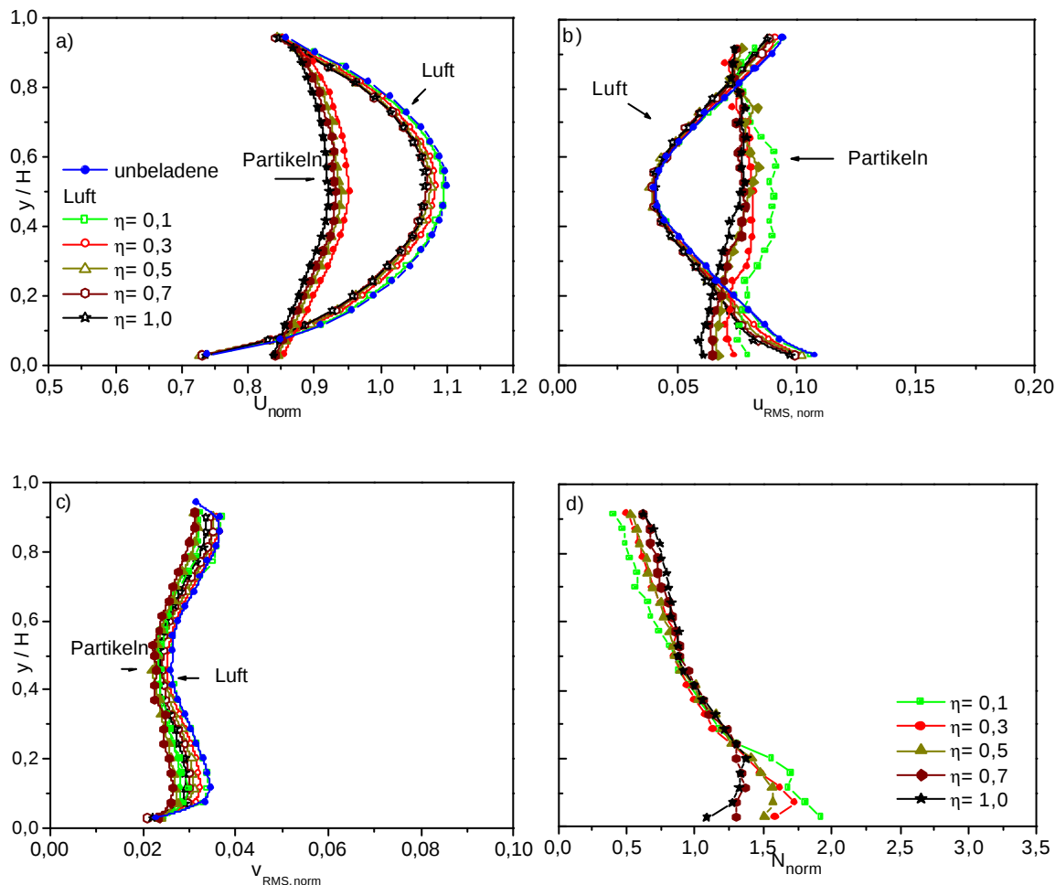
Abbildung 5-27: Normierte Profile der Luft und der 487µm zylindrischen Polycarbonatpartikeln bei einem U_{\text{mittel}} von 19,95 m/s und der Wandrauhigkeit R0: a) horizontale Geschwindigkeit der Luft und der Partikeln, b) RMS- Profil der horizontalen Komponenten, c) RMS- Profil der vertikalen Komponenten, d) vertikale Sampleverteilung der Partikeln. Die gefüllten Symbole stellen jeweils die Feststoffphase, die leeren Symbole die Gasphase dar.
