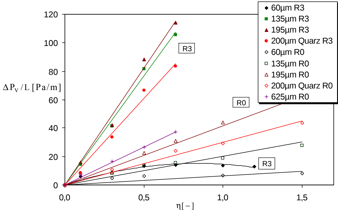
Abbildung 5-47: Resultierende Druckverlust in Abhängigkeit von der Beladung für eine glatte Wand R0 und einer rauhen Wand R3, sphärische Glas- und nichtsphärische Quarzpartikeln, U_{\text{mittel}} = 20 \text{ m/s} .
