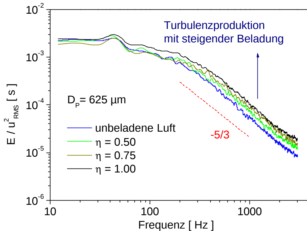
Abbildung 5-39: Energiespektrum der horizontalen Geschwindigkeitskomponente im Zentrum des Kanals bei verschiedenen Feststoffbeladungen ( U_{\text{mittel}} = 19,1 \text{ m/s} , Wandrauhigkeit R1, D_p = 625 \mu\text{m} ).
