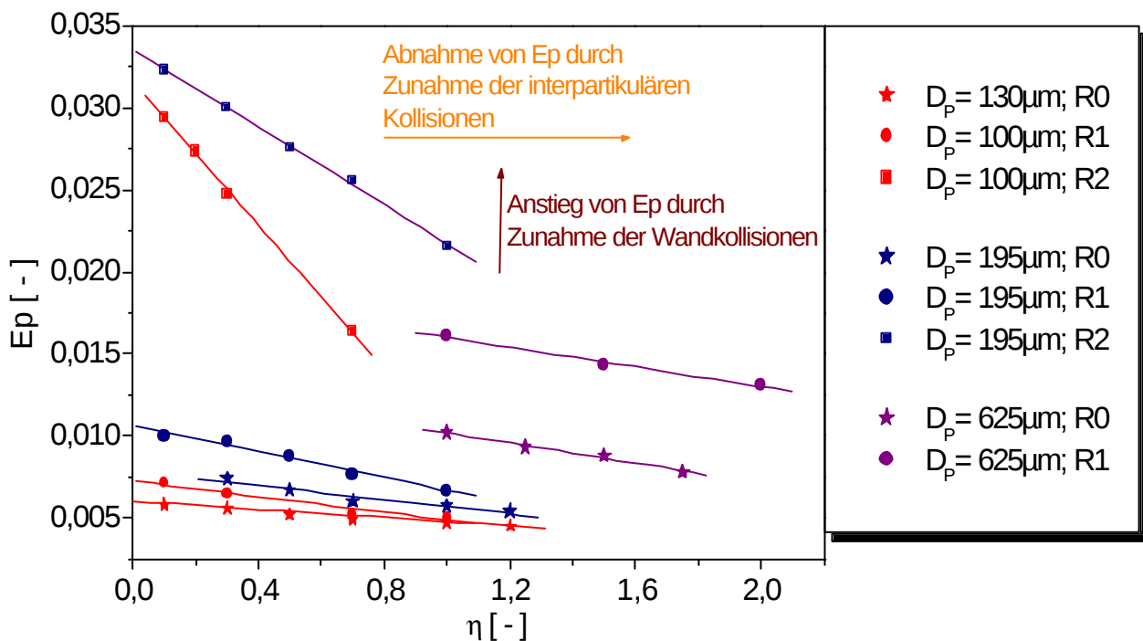
Abbildung 5-24: Normalisierte Energie der Partikelschwankungsgeschwindigkeit in Abhängigkeit von der Beladung für unterschiedliche Partikelgrößen und Wandrauhigkeiten. U_{\text{mittel}} zwischen 19,7 und 20,2 m/s.
