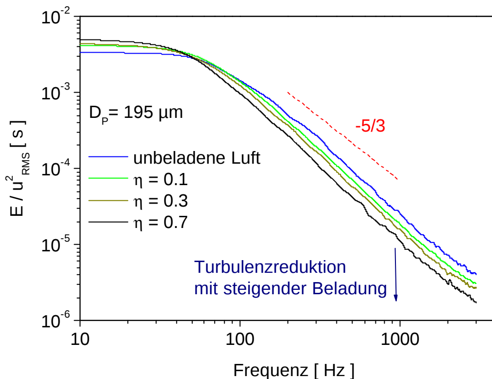
Abbildung 5-38: Energiespektrum der horizontalen Geschwindigkeitskomponente im Zentrum des Kanals bei verschiedenen Feststoffbeladungen ( U_{\text{mittel}}=19,7 m/s, Wandrauhigkeit R1, D_p=195\mu\text{m} ).
