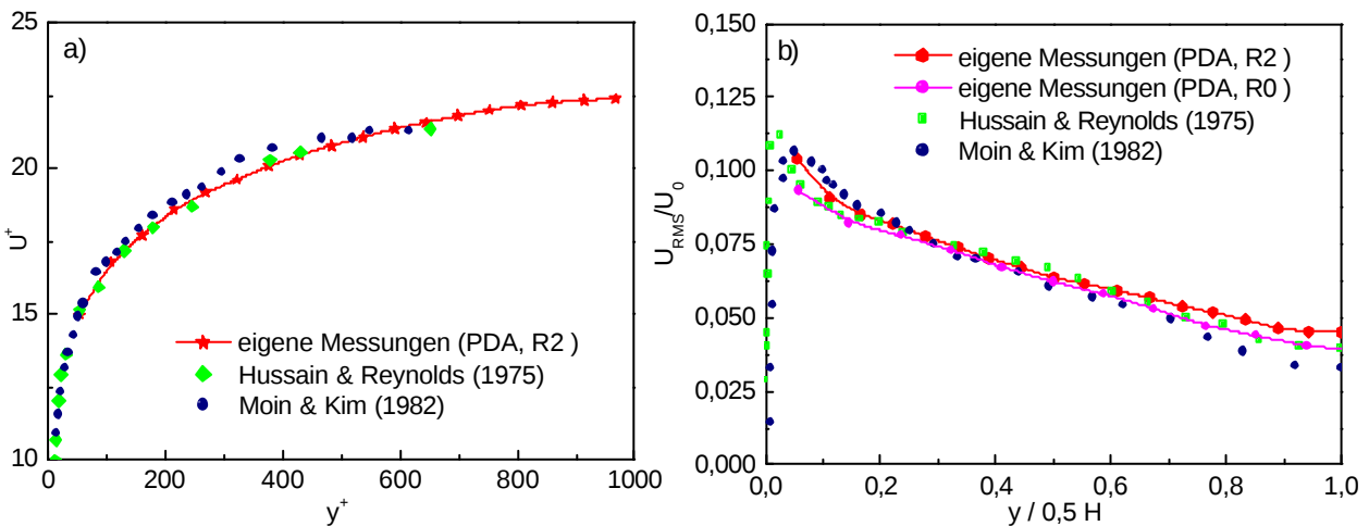
Abbildung 5-3: a-b) Vergleich der normierten Ein- Phasenströmung mit Messungen von HUSSAIN und REYNOLDS [25] sowie mit LES- Daten von MOIN und KIM [37] a) horizontale Geschwindigkeit und b) horizontale Schwankungsgeschwindigkeit.
