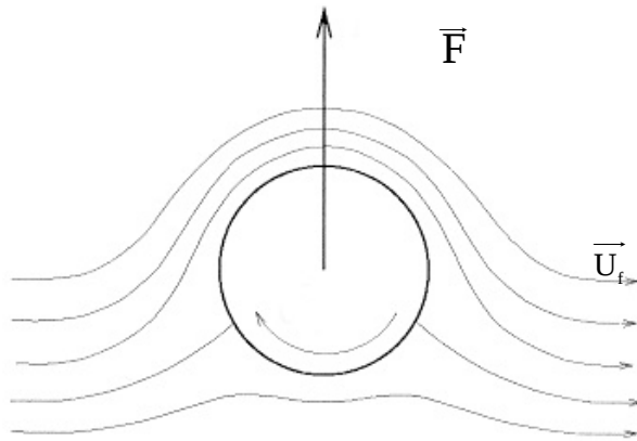
Abbildung 3-8: Prinzip des Magnus-Effekt: Durch die Rotation des Partikels folgt eine unsymmetrische Umströmung, so dass eine Kraft in Richtung der höchsten Umströmgeschwindigkeit folgt
