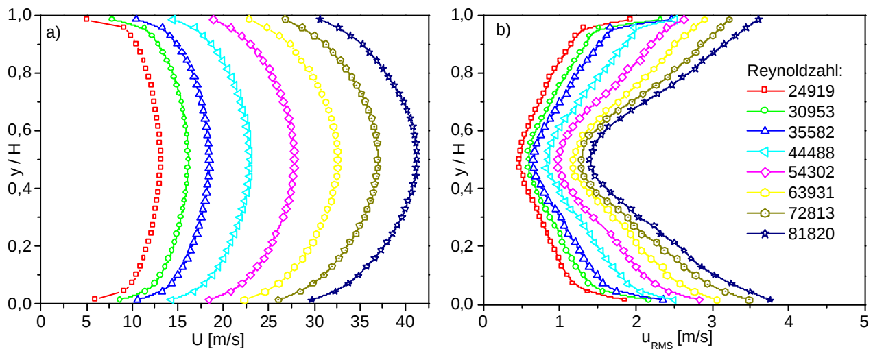
Abbildung 5-1: Vertikale Profile der a) horizontalen Geschwindigkeit und b) der horizontalen Schwankungsgeschwindigkeit bei unterschiedlichen Reynolds- Zahlen, Wandrauhigkeit R2.
