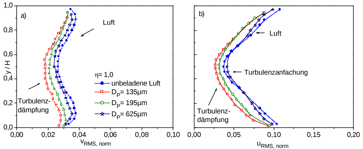
Abbildung 5-22: Normierte a) vertikale und b) horizontale Profile der Luft ( U_{\text{mittel}} von 20,2 m/s bei 135 und 195 \mu\text{m} - Partikeln und 20,1 m/s bei 625 \mu\text{m} ) bei einer Beladung von 1,0 für unterschiedliche Partikelgrößen, Wandrauigkeit R0.
