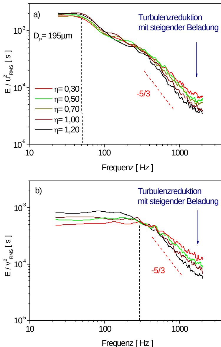
Abbildung 5-41: Energiespektren der a) horizontalen und b) der vertikalen Geschwindigkeitskomponenten. D_p = 195\mu\text{m} , Wandrauhigkeit R0, U_{\text{mittel}} = 20,2 \text{ m/s} .
