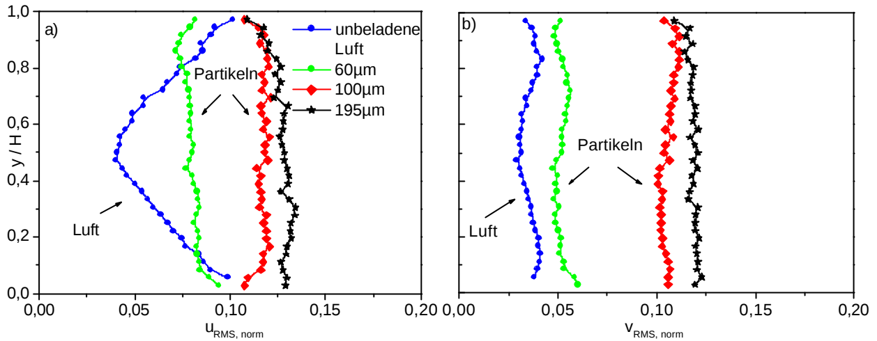
Abbildung 5-17: Normierte vertikale Profile der a) horizontalen und b) vertikalen Schwankungsbewegung der Partikel für unterschiedliche Größen, Wandrauhigkeit R2, Beladung \eta = 0,3 (60µm \eta = 0,2 ), U_{mittel} = 19,7 m/s.
