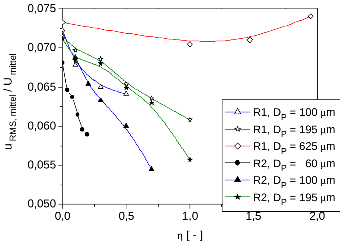
Abbildung 5-42: Über die Kanalhöhe normalisierte horizontale Schwankungsgeschwindigkeit der Luft in Abhängigkeit von der Beladung, der Wandrauhigkeit R1 und R2, und der Partikelgröße ( U_{\text{mittel, Kanalzentrum}} \approx 21 \text{ m/s} ).
