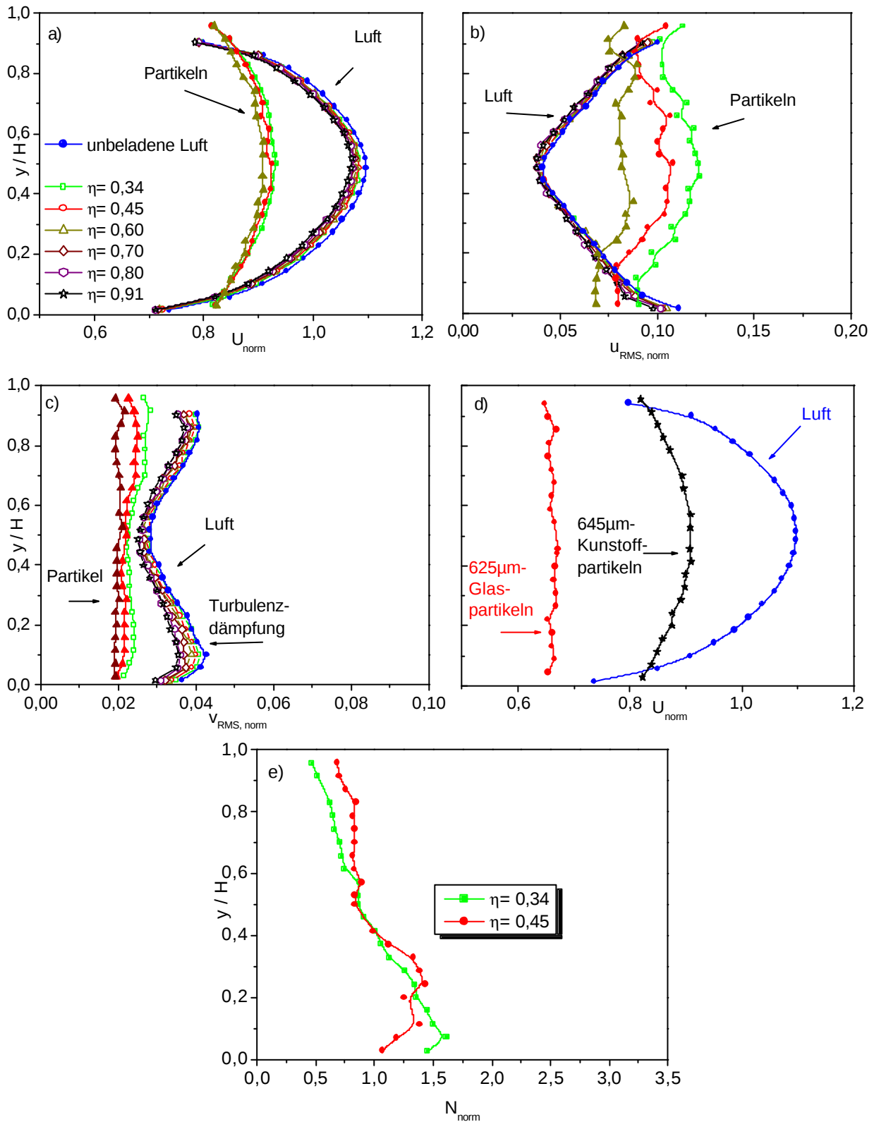
Abbildung 5-23: a-d) Normierte Profile der Luft und der 645µm- Polystyrolpartikeln bei einem U_{\text{mittel}} von 20,3 m/s und der Wandrauigkeit R0: a) horizontale Geschwindigkeit der Luft und der Partikeln, b) RMS- Profil der horizontalen Komponente, c) RMS- Profil der vertikalen Komponente, d) Vergleich der normierten horizontalen Partikelgeschwindigkeit der 625µm Glaspartikeln ( \eta = 0,7 , U_{\text{mittel}} = 20,1 m/s) und 645µm Polystyrolpartikeln ( \eta = 0,6 ), e) vertikales Profil der normierten Samplekonzentration. Die gefüllten Symbole stellen jeweils die Feststoffphase, die leeren Symbole die Gasphase dar.
