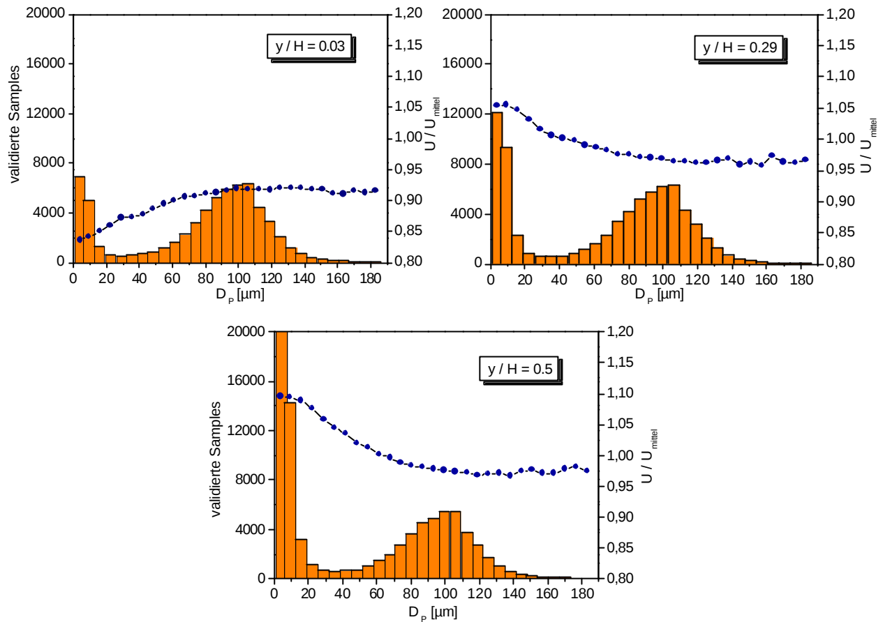
Abbildung 4-17: Größenverteilung der Tracer und der Partikeln (vertikale Balken), zusammen mit der Größen- Geschwindigkeitskorrelation (Linie mit Symbol): a) y / H = 0,03 Kanalboden, b) y / H = 0,29 , c) y / H = 0,5 Kanalmitte ( U_{\text{mittel}} = 19,7 \text{ m/s} , 100 \mu\text{m} Glaspartikeln, \eta = 0,3 , Rauigkeit R1, y / H = normierter Wandabstand).
