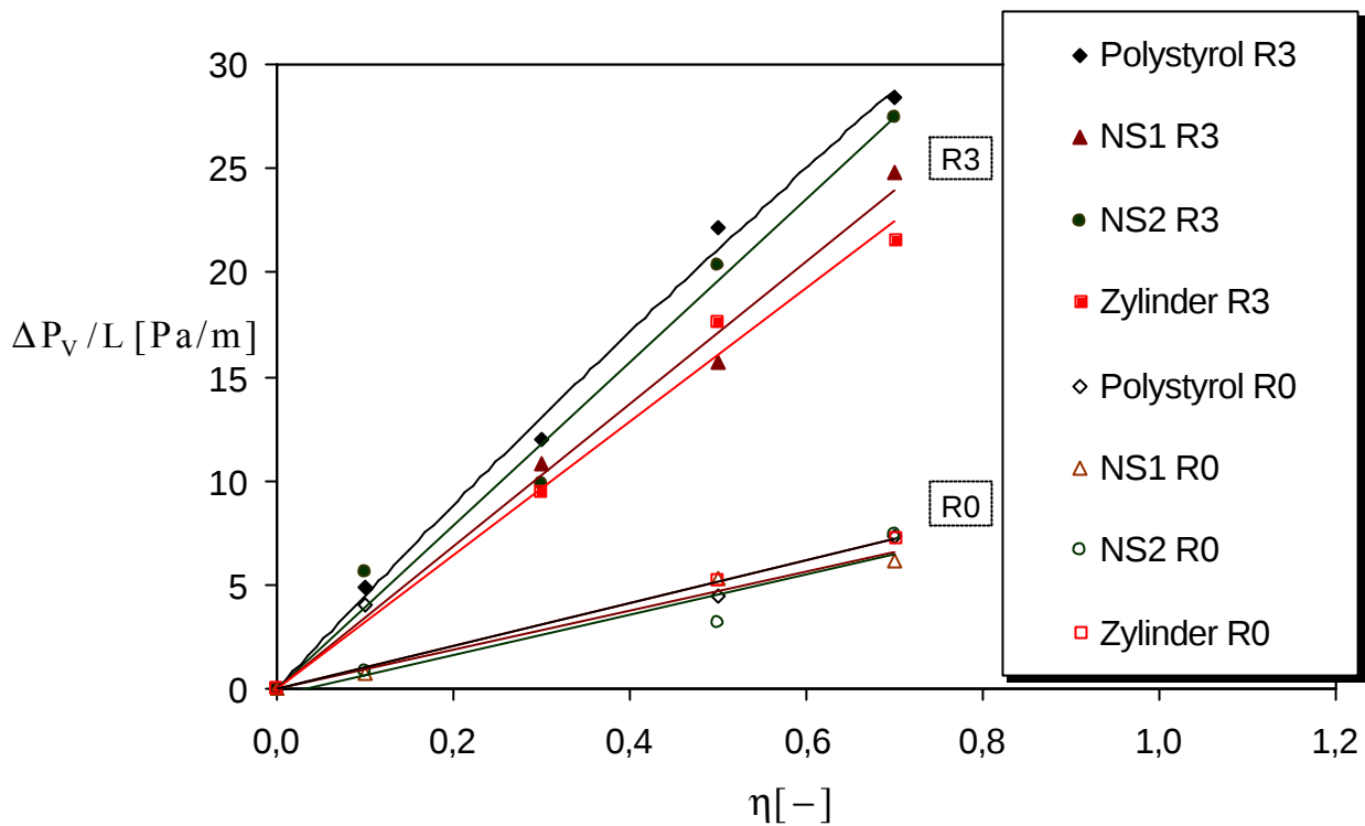
Abbildung 5-48: Resultierende normierter Druckverlust in Abhängigkeit von der Beladung für eine glatte Wand R0 und einer rauen Wand R3, sphärische und nichtsphärische Kunststoffpartikeln, U_{\text{mittel}} = 20 \text{ m/s} .
