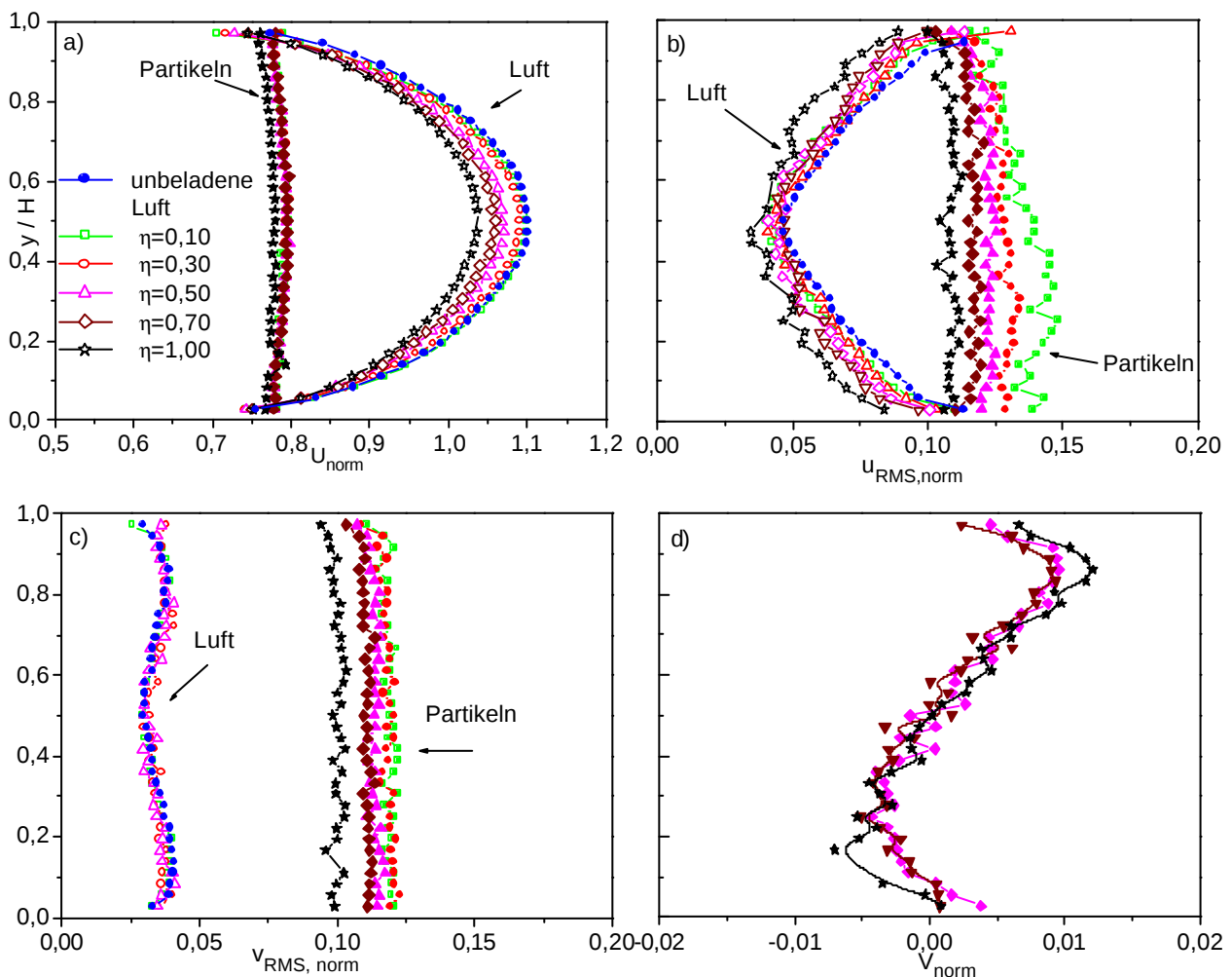
Abbildung 5-14: a-c) Normierte Profile der Luft und der 195\mu\text{m} - Partikeln bei einem U_{\text{mittel}} von 19,7 m/s und der Wandrauhigkeit R2: a) horizontale Geschwindigkeit der Luft und der Partikeln, b) RMS- Profil der horizontalen Komponente, c) RMS- Profil der vertikalen Komponente, d) Profil der normierten vertikalen Anzahlkonzentration der Partikeln. Die gefüllten Symbole stellen jeweils die Feststoffphase, die leeren Symbole die Gasphase dar.
