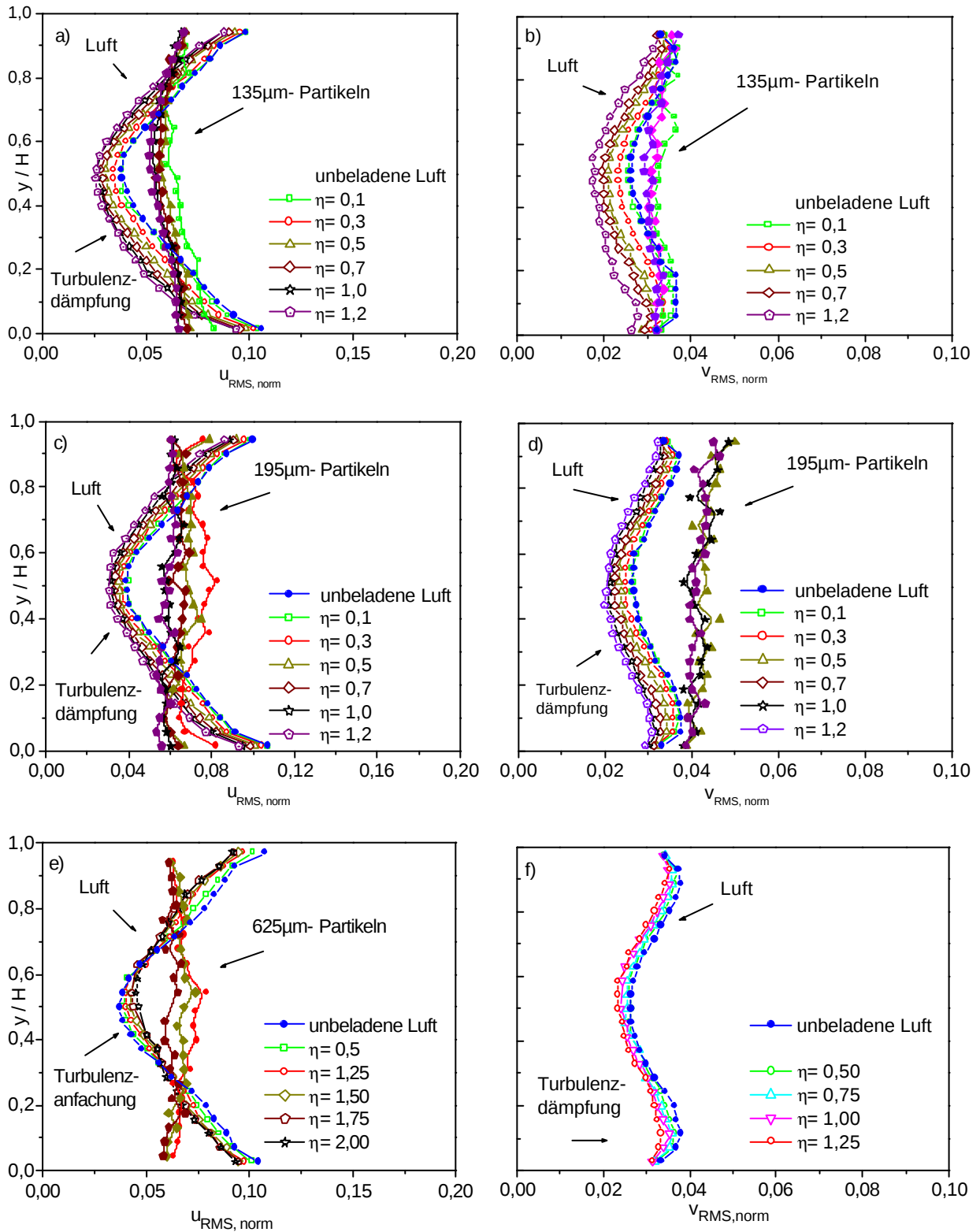
Abbildung 5-21: a und f) Normierte Profile der Luft und der Partikel bei einem U_{mittel} von 20,2 m/s (135 und 195µm) und 20,1m/s (625µm), Wandrauhigkeit R0; a, c und e) normierte horizontale Schwankungsgeschwindigkeit; b, d und f) normierte vertikale Schwankungsgeschwindigkeit. Die vertikale Schwankungsgeschwindigkeit der 625µm- Partikeln konnte wegen messtechnischen Begrenzungen nicht erfasst werden. Die gefüllten Symbole stellen jeweils die Feststoffphase, die leeren Symbole die Gasphase dar.
