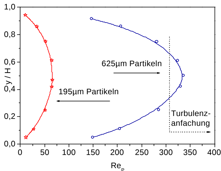
Abbildung 5-8: Vertikale Profile der Partikel-Reynoldszahl für zwei verschiedene Partikelgrößen bei einer Massenbeladung von 1.0 und einer Wandrauhigkeit R1.
