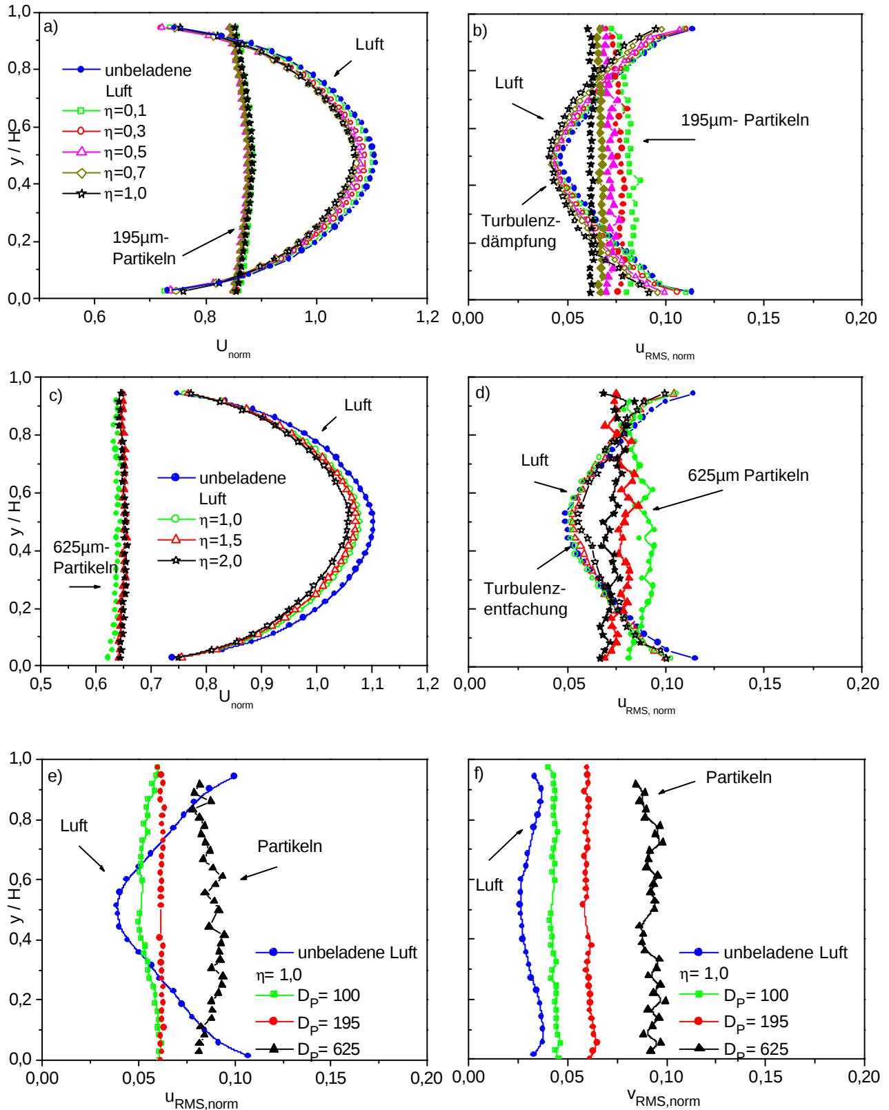
Abbildung 5-6: a-f) Normierte vertikale Profile der Luft und der Partikeln bei einem U_{\text{mittel}} von 19,7 m/s (100µm und 195µm) und 19,1m/s (625µm), Wandrauhigkeit R1: a und c) horizontale Geschwindigkeit der Luft und der Partikeln, (b und d) u_{\text{RMS}} - Profil der Luft und der Partikeln, e) Vergleich der Partikel u_{\text{RMS}} - Profile unterschiedlicher Größen, f) Vergleich der Partikel v_{\text{RMS}} - Profile unterschiedlicher Größen. Die gefüllten Symbole stellen jeweils die Feststoffphase, die leeren Symbole die Gasphase dar.
