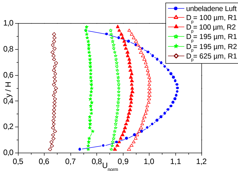
Abbildung 5-15: Normiertes vertikales Profil der horizontalen Geschwindigkeitskomponente der Feststoffphase bei unterschiedlich großen Partikeln und Wandrauhigkeiten R1 und R2. U_{\text{mittel}} = 19,7\ \text{m/s} , \eta = 1 .
