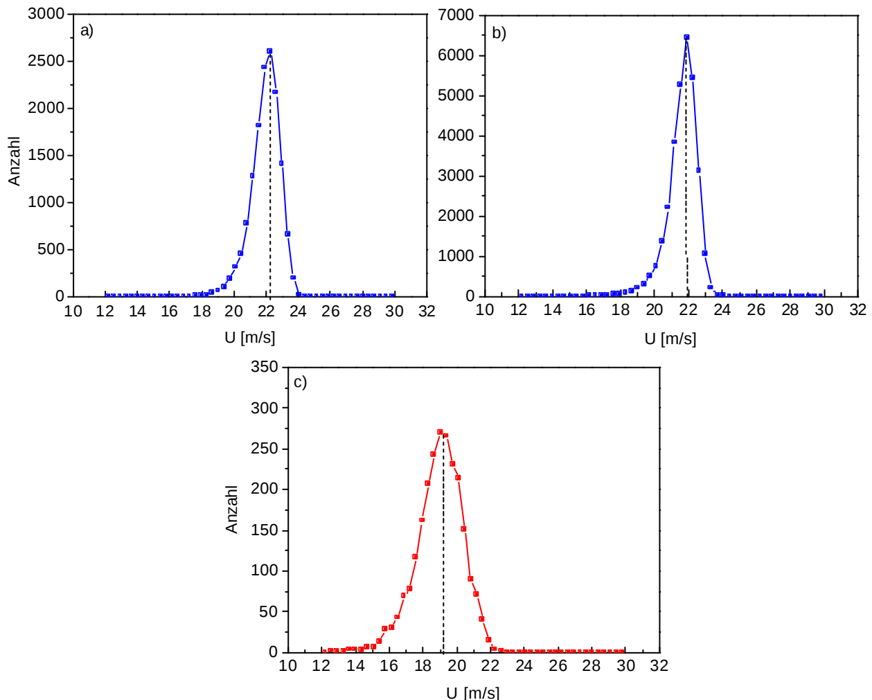
Abbildung 4-19: Anzahl- Geschwindigkeitsverteilung a) der Tracer bei \eta=0 , b) Tracer bei \eta=0,3 und c) der Quarzpartikeln bei \eta=0,3 und einer Wandrauhigkeit R_0 in der Mitte des Kanals, U_{\text{mittel}} = 20,1 m/s.
