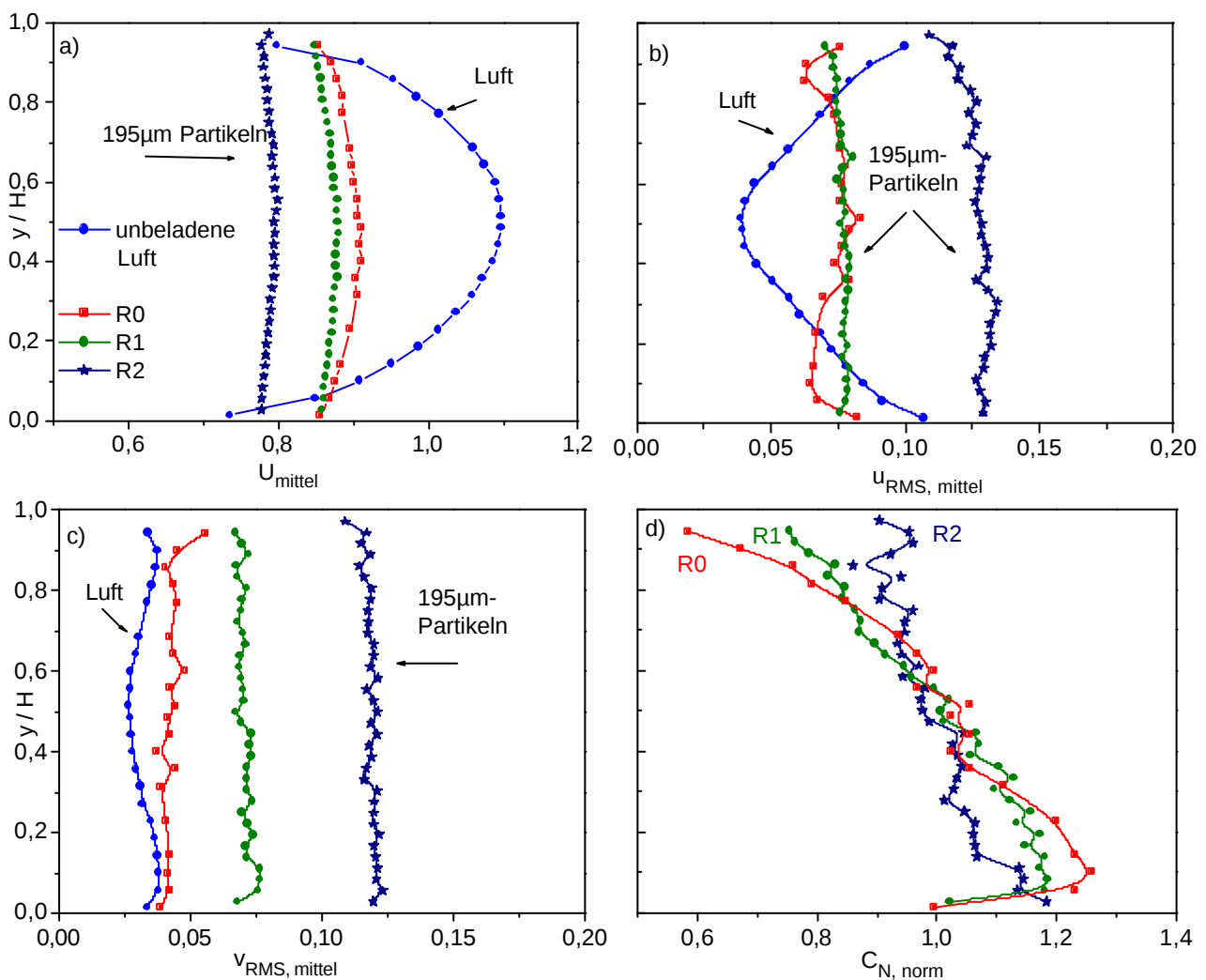
Abbildung 5-19: a-c) Normierte Profile der 195\ \mu\text{m} - Partikeln bei einem U_{\text{mittel}} von 19,7 (R1 und R2) und 20,2\ \text{m/s} (R0) und unterschiedlichen Wandrauigkeiten R0, R1 und R2, \eta=0,3 : a) horizontale Geschwindigkeit der Partikeln, b) Partikel- RMS- Profil der horizontalen Komponente, c) Partikel- RMS- Profil der vertikalen Komponente, d) Profil der normierten vertikalen Anzahlkonzentration der Partikeln. Die gefüllten Symbole stellen jeweils die Feststoffphase, die leeren Symbole die Gasphase dar.
