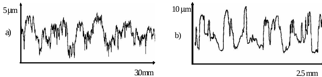
Abbildung 4-2: Gemessene Rauigkeitsprofile bei zwei unterschiedlichen Edelstahlplatten: a) R1 geringe Rauigkeit, b) R2 höhere Rauigkeit
