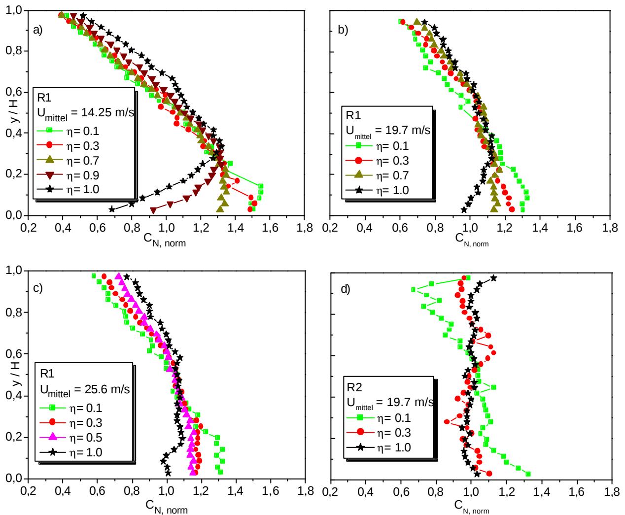
Abbildung 5-11: a-d) Normiertes vertikales Profil der normalisierten Partikelkonzentration ( D_p = 100\mu\text{m} ) bei unterschiedlichen Bedingungen a) Rauigkeit R1 und U_{\text{mittel}} = 14,25 \text{ m/s} , b) Rauigkeit R1 und U_{\text{mittel}} = 19,70 \text{ m/s} , c) Rauigkeit R1 und U_{\text{mittel}} = 25,60 \text{ m/s} und d) Rauigkeit R2 und U_{\text{mittel}} = 19,70 \text{ m/s} .
