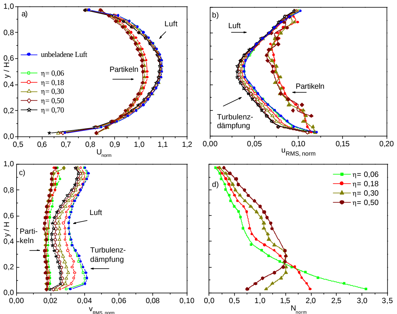
Abbildung 5-25: Normierte Profile der Luft und der 185µm Duroplastpartikeln I bei einem U_{\text{mittel}} von 19,8 m/s und der Wandrauhigkeit R0: a) horizontale Geschwindigkeit der Luft und der Partikeln, b) RMS- Profil der horizontalen Komponenten, c) RMS- Profil der vertikalen Komponenten, d) vertikale Sampleverteilung der Partikeln. Die gefüllten Symbole stellen jeweils die Feststoffphase, die leeren Symbole die Gasphase dar.
