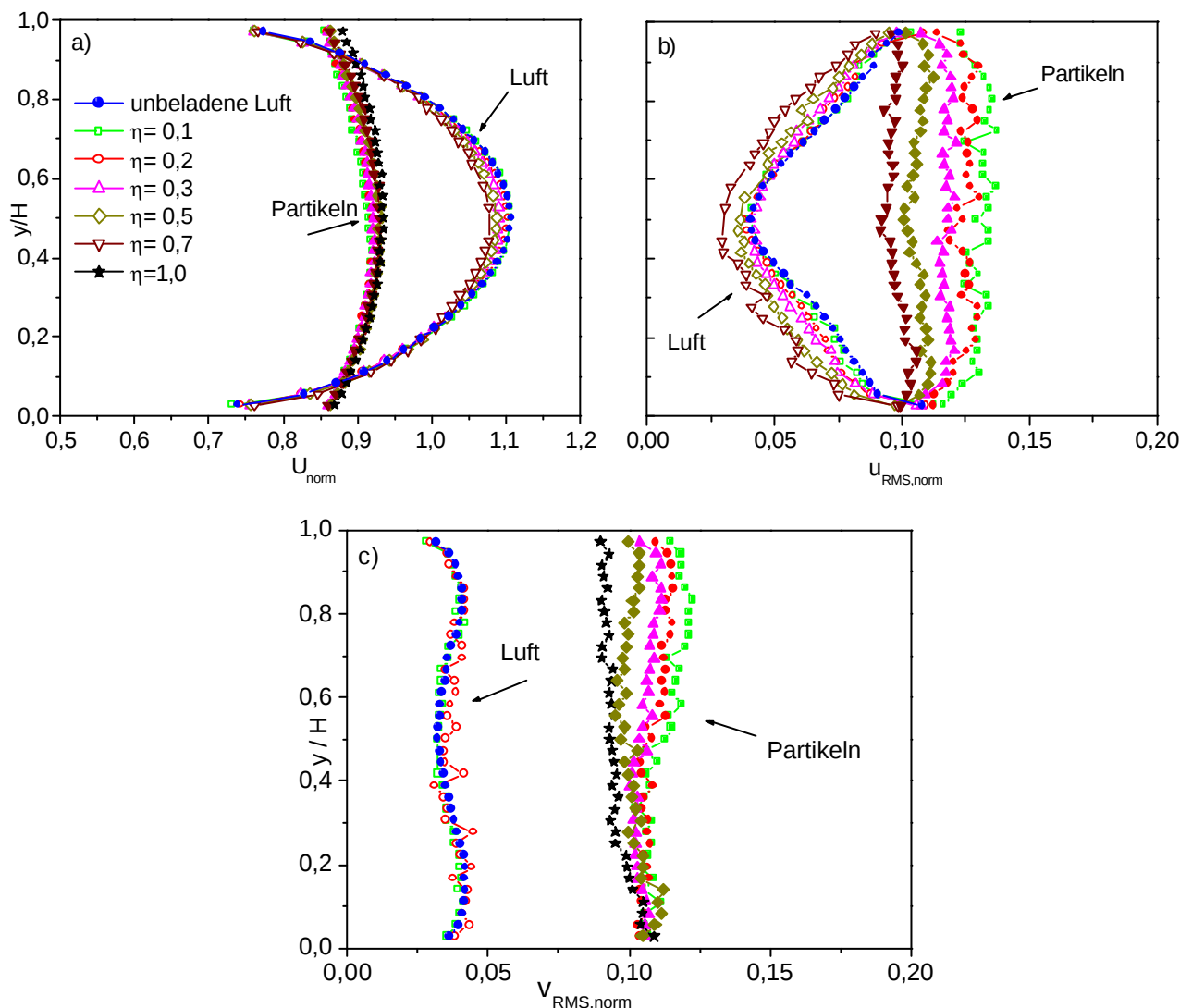
Abbildung 5-9: a-c) Normierte Profile der Luft und der 100 \mu m- Partikeln bei einem U_{\text{mittel}} von 19,7 m/s und der Wandrauhigkeit R2: a) horizontale Geschwindigkeit der Luft und der Partikeln, b) RMS- Profile der horizontalen Komponenten, c) RMS- Profile der vertikalen Komponenten. Die gefüllten Symbole stellen jeweils die Feststoffphase, die leeren Symbole die Gasphase dar.
