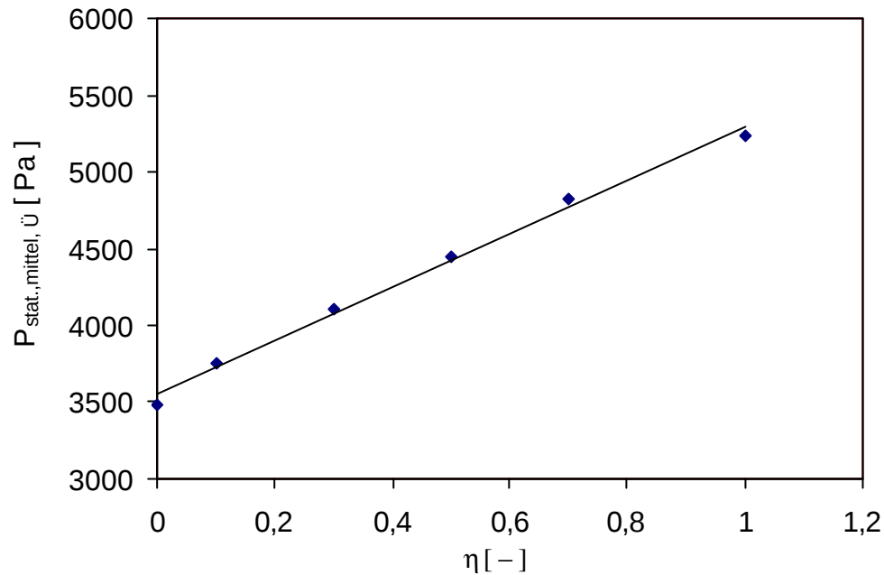
Abbildung 5-44: Mittlerer statischer Überdruck in Abhängigkeit von der Beladung, Wandrauhigkeit R0, D_p = 195\mu\text{m} - Glaspartikeln, U_{\text{mittel}} = 20 \text{ m/s} .
