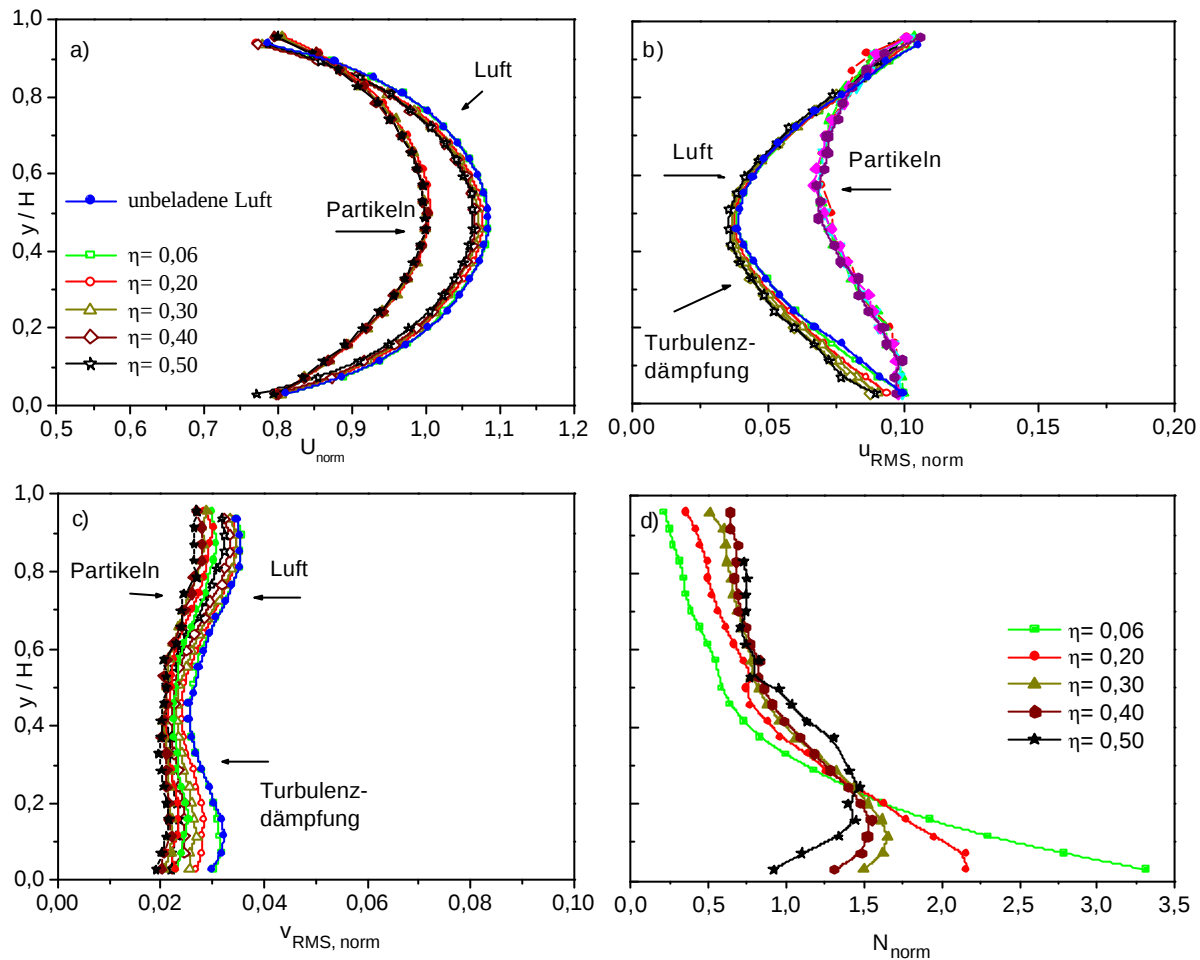
Abbildung 5-26: Normierte Profile der Luft und der 245µm Duroplastpartikeln II bei einem U_{\text{mittel}} von 20,4 m/s und der Wandrauhigkeit R_0 : a) horizontale Geschwindigkeit der Luft und der Partikel, b) RMS- Profil der horizontalen Komponenten, c) RMS- Profil der vertikalen Komponenten, d) vertikale Sampleverteilung der Partikeln. Die gefüllten Symbole stellen jeweils die Feststoffphase, die leeren Symbole die Gasphase dar.
